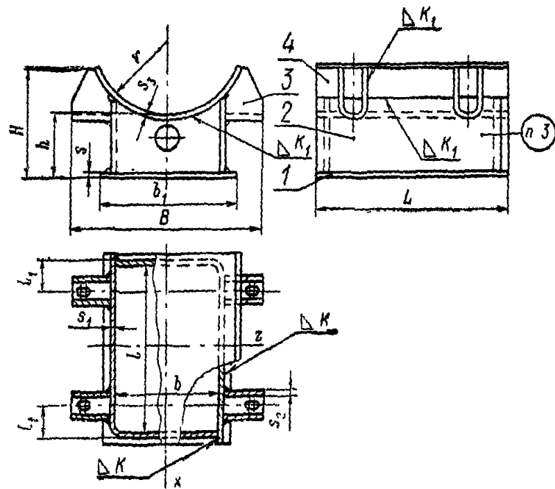
1 — основание; 2 — угольник; 3 — прошина; 4 — подушка
